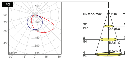
P2 + BARRA/STRIP/3E + 70092/C
