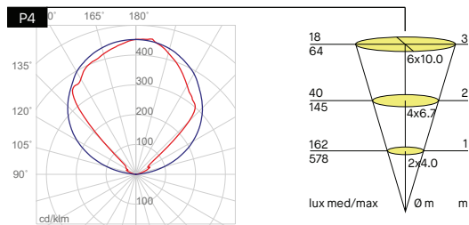
P4 + BARRA/STRIP/3E + 70092/C
